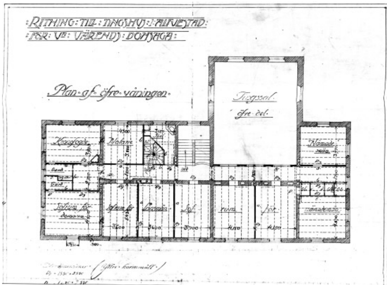
Planritning av tingshusets övervåning upprättad av arkitektfirma Ewe & Melin år 1905.
