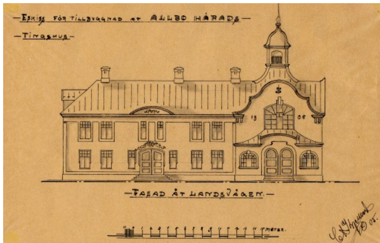
Ombyggnadsförslag för gamla tingshuset i Alvesta upprättat 1905 före beslut togs att låta uppföra en helt ny tingshusbyggnad. Skissen hämtad ur Tingshusbyggnadsskyldiges vid Västra Väreuds domsaga arkiv volym Ö:2, Vadstena Landsarkiv.
