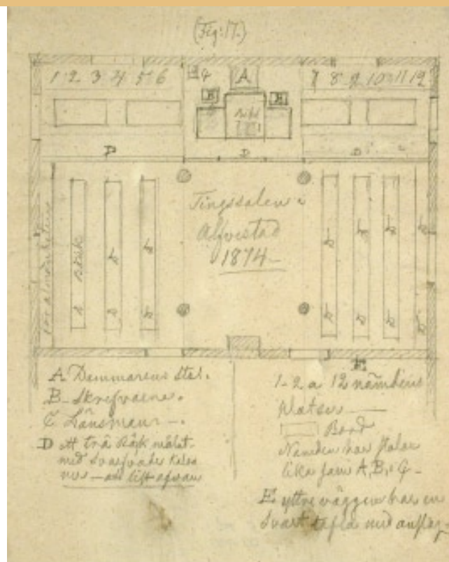
Skiss över tingsalen i det gamla tingshuset upprättad av Nils Månsson Mandelgren. Huset slutade brukas som tingshus sedan det nya tingshuset stod klart år 1907. Det gamla tingshuset stod sedan kvar som privatbostad fram till år 1967 då huset revs. Enligt uppgift från en tidigare hyresgäst skall tingsalen ha byggts om till lägenhet med bland annat en kakelugn som värmekälla. Skiss hämtad ur Mandelgrenska samlingen, Folklivsarkivet Lund.
