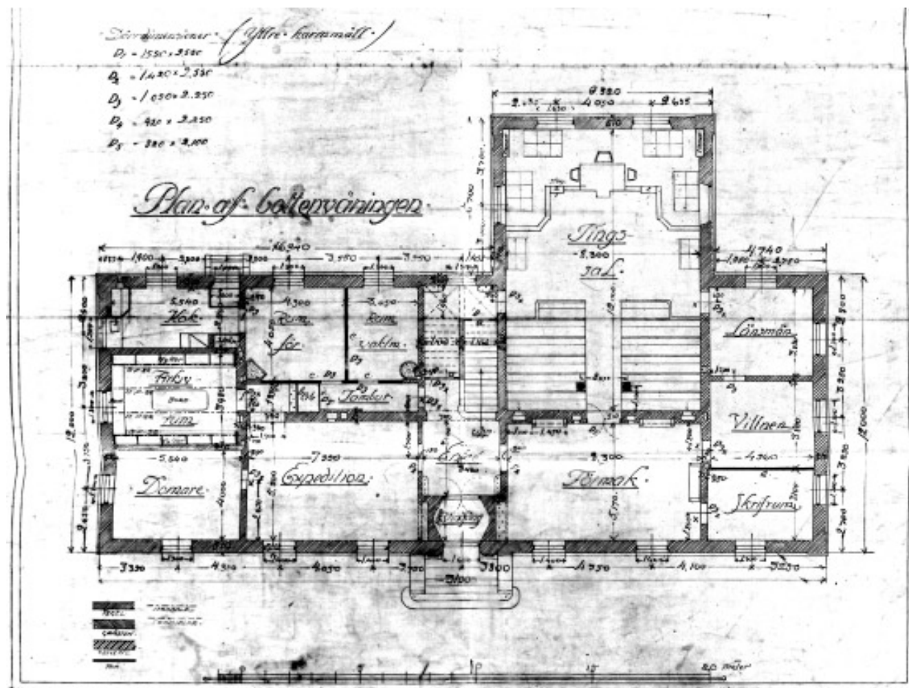
Planritning av tingshusets bottenvåning upprättad av arkitektfirma Ewe & Melin år 1905.
